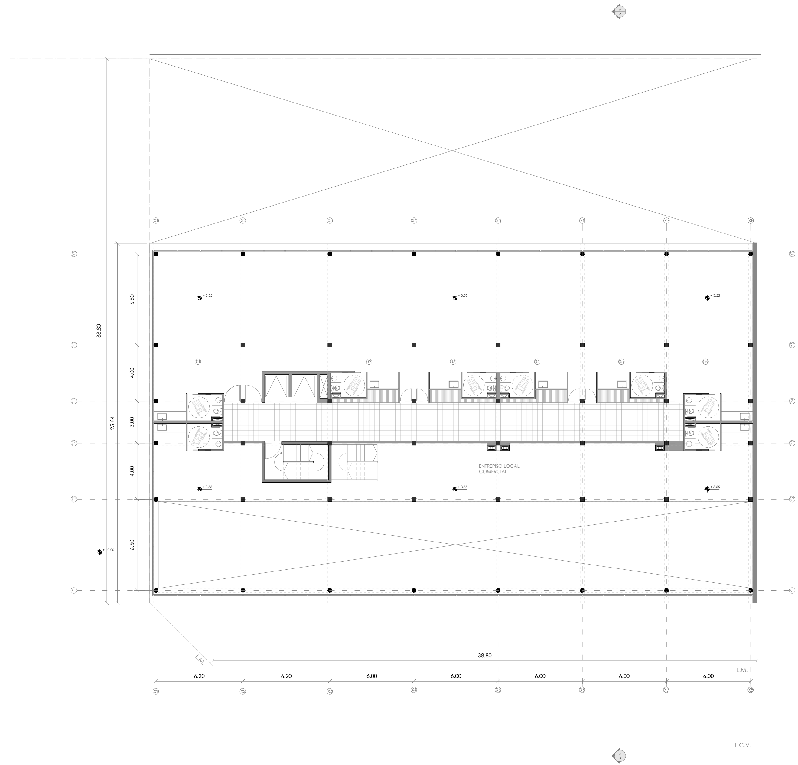
PLANTA PRIMER PISO
